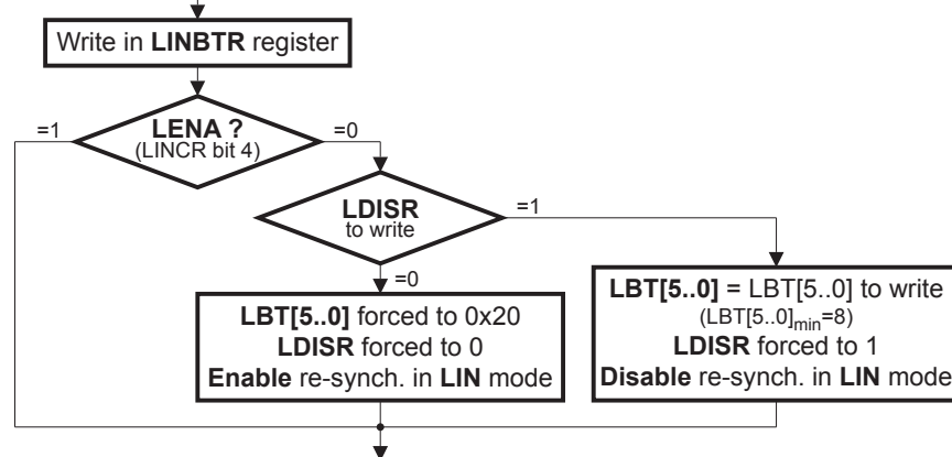
Figure 21-8. Handling LBT[5:0].
